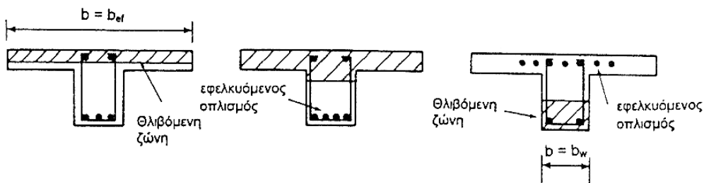
(b) Διατομή A - A (ορθογωνική θλιβόμενη ζώνη)
