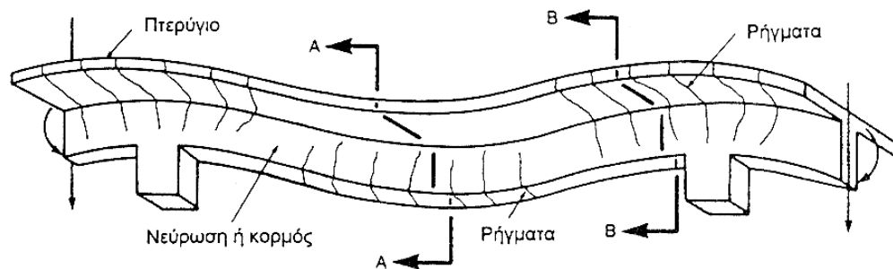
(a) Παραμορφωμένη δοκός
